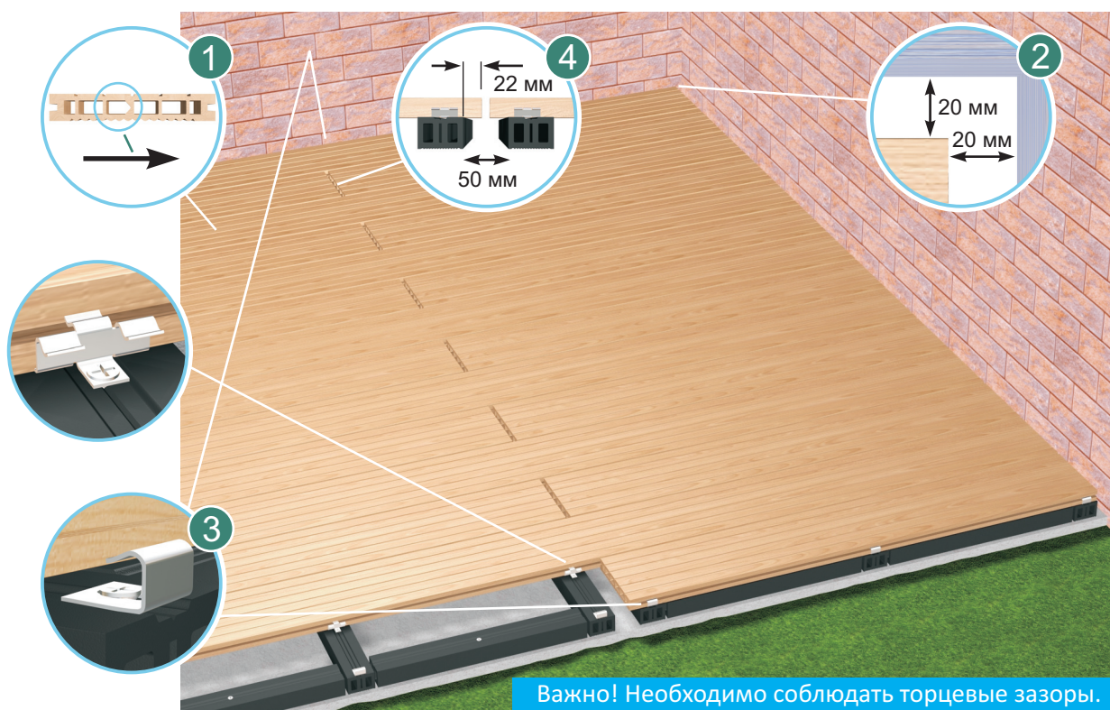
Торцевые зазоры для монтажа досок, мм
